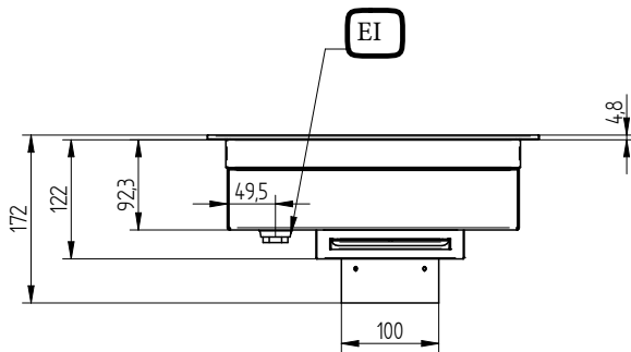
Alzado
